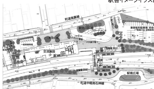
橋上駅舎・自由通路周辺図面
