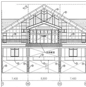
北側立面図
